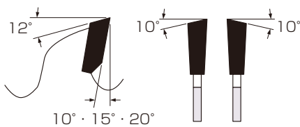
■BC交互リード刃型 BC-ATB (Alternative Top Bevel)
